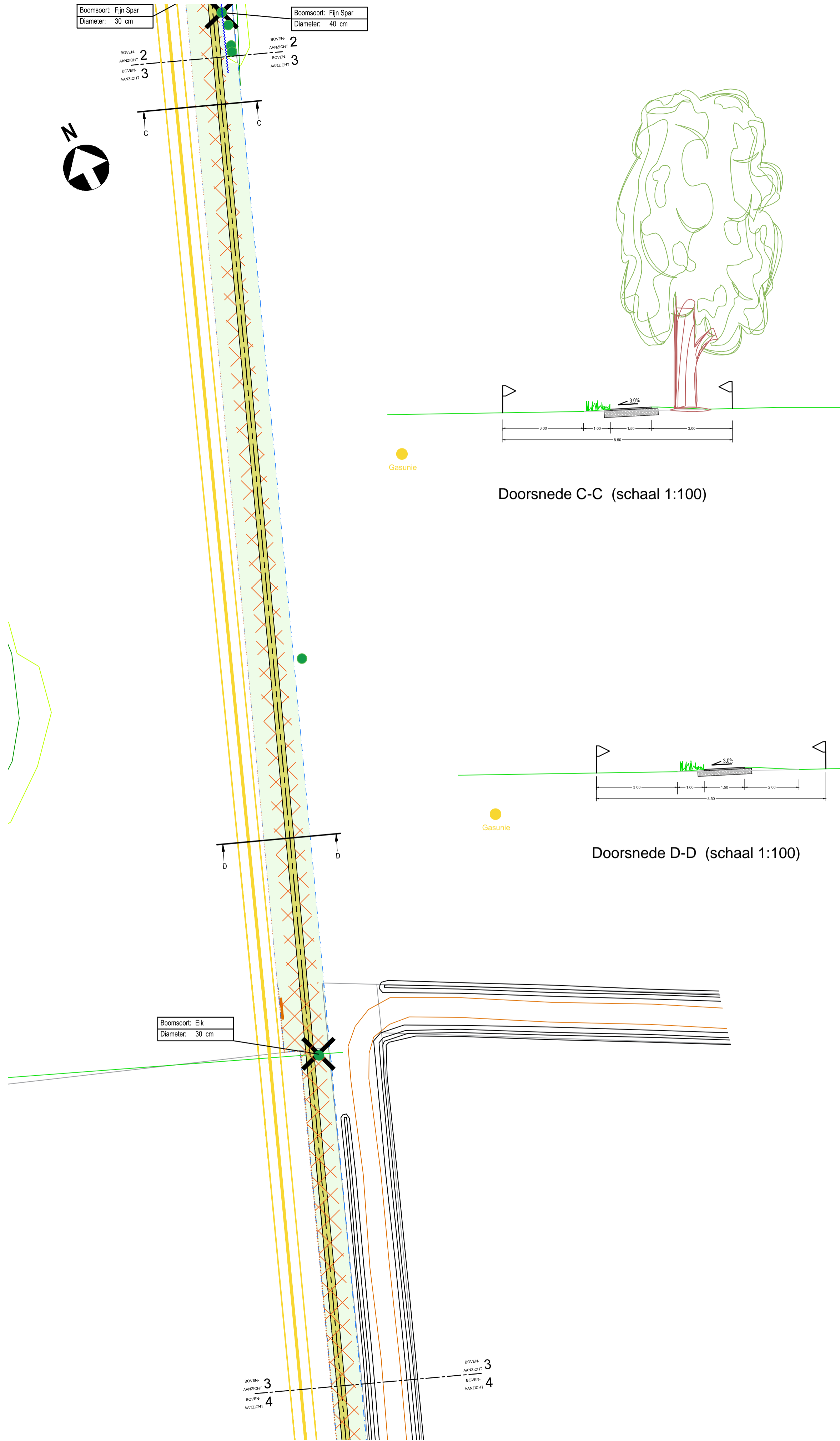
Bovenaanzicht 3 (schaal 1:500)
