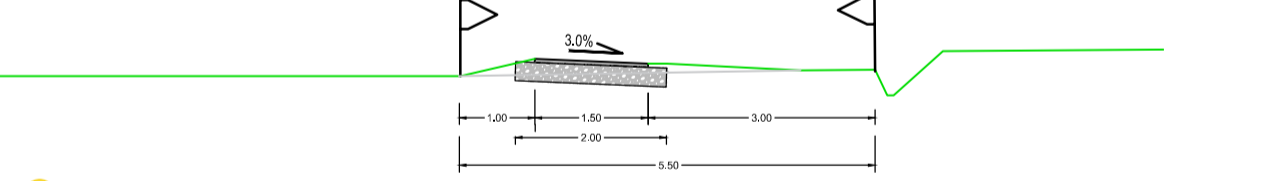
Doorsnede E-E (schaal 1:100)
