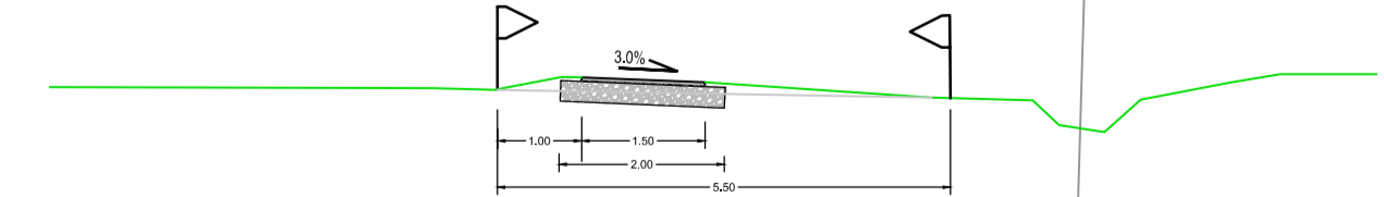
Doorsnede F-F (schaal 1:100)
