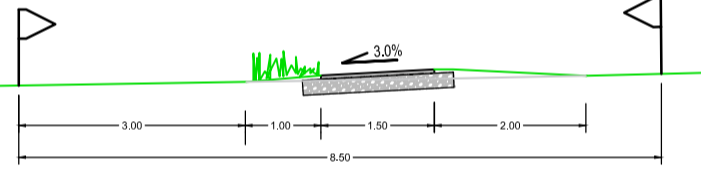
Doorsnede D-D (schaal 1:100)
