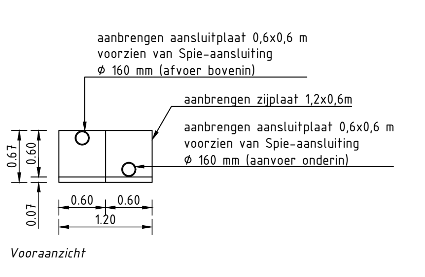
Detail infiltratie kratten Q-Bic Plus Schaal 1:50
