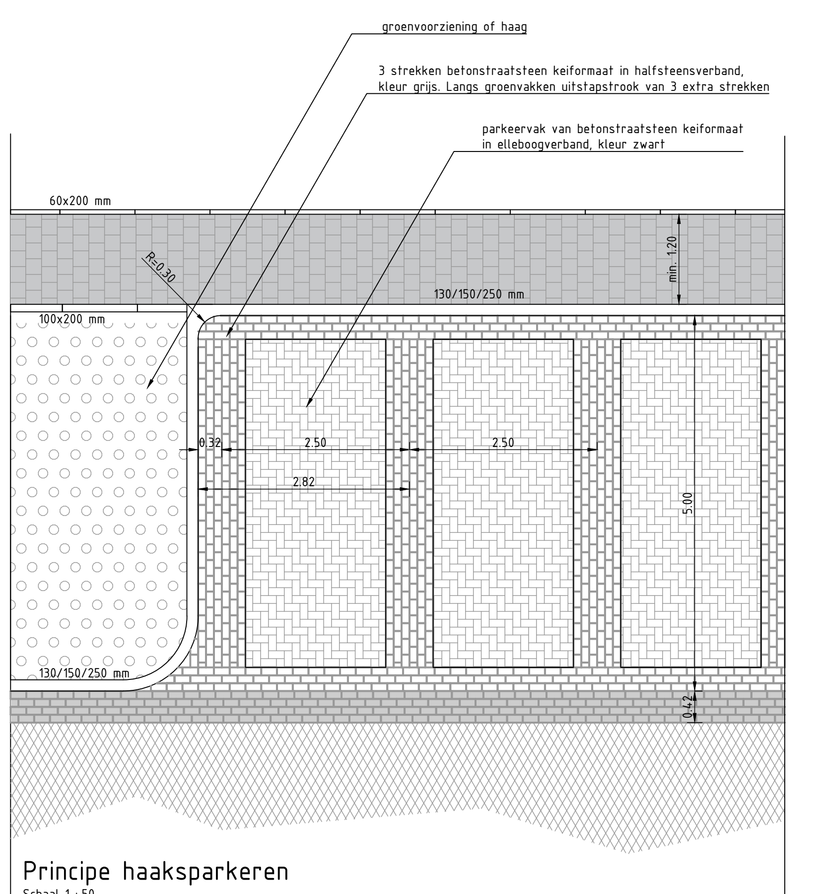
Principe haaksparkeren Schaal 1:50
