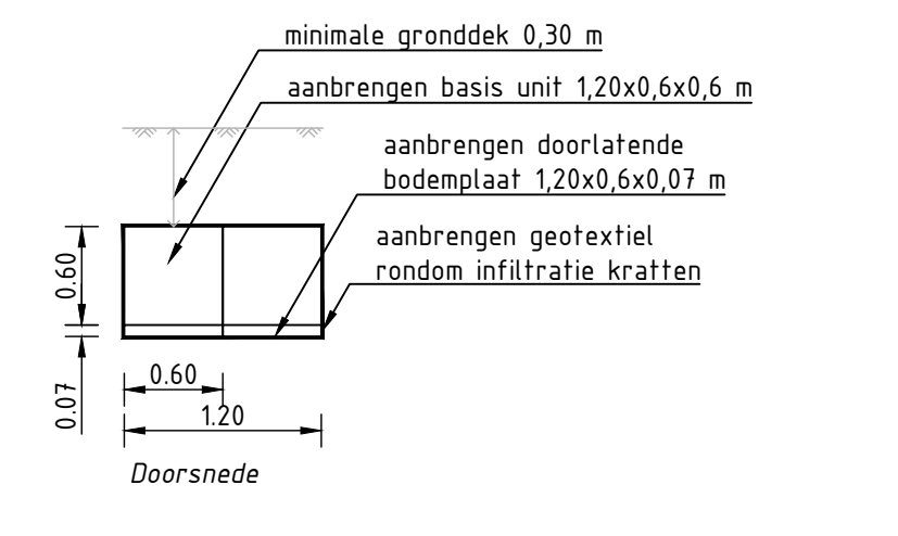
Profiel A-A Schaal 1:50
