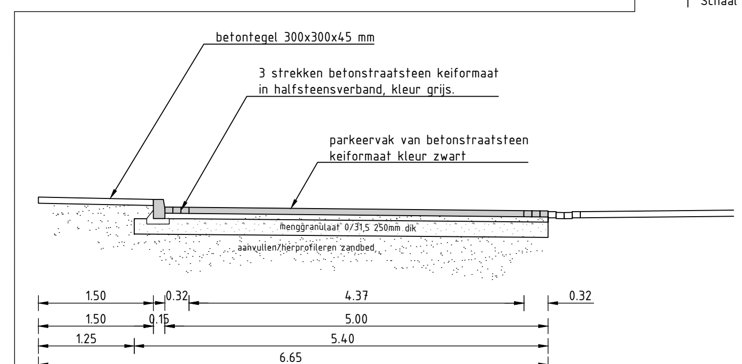
Fundatie parkeren Schaal 1:50
