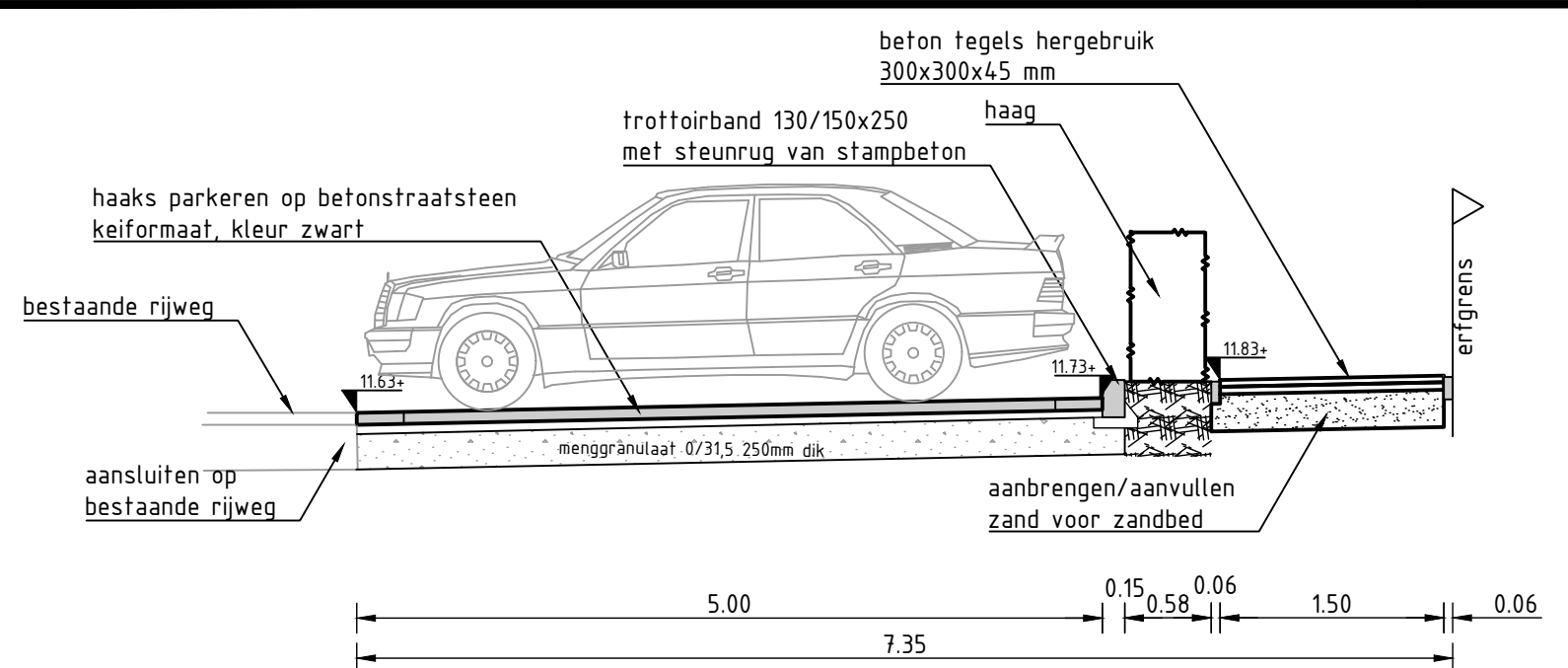
Profiel A-A Schaal 1:50
