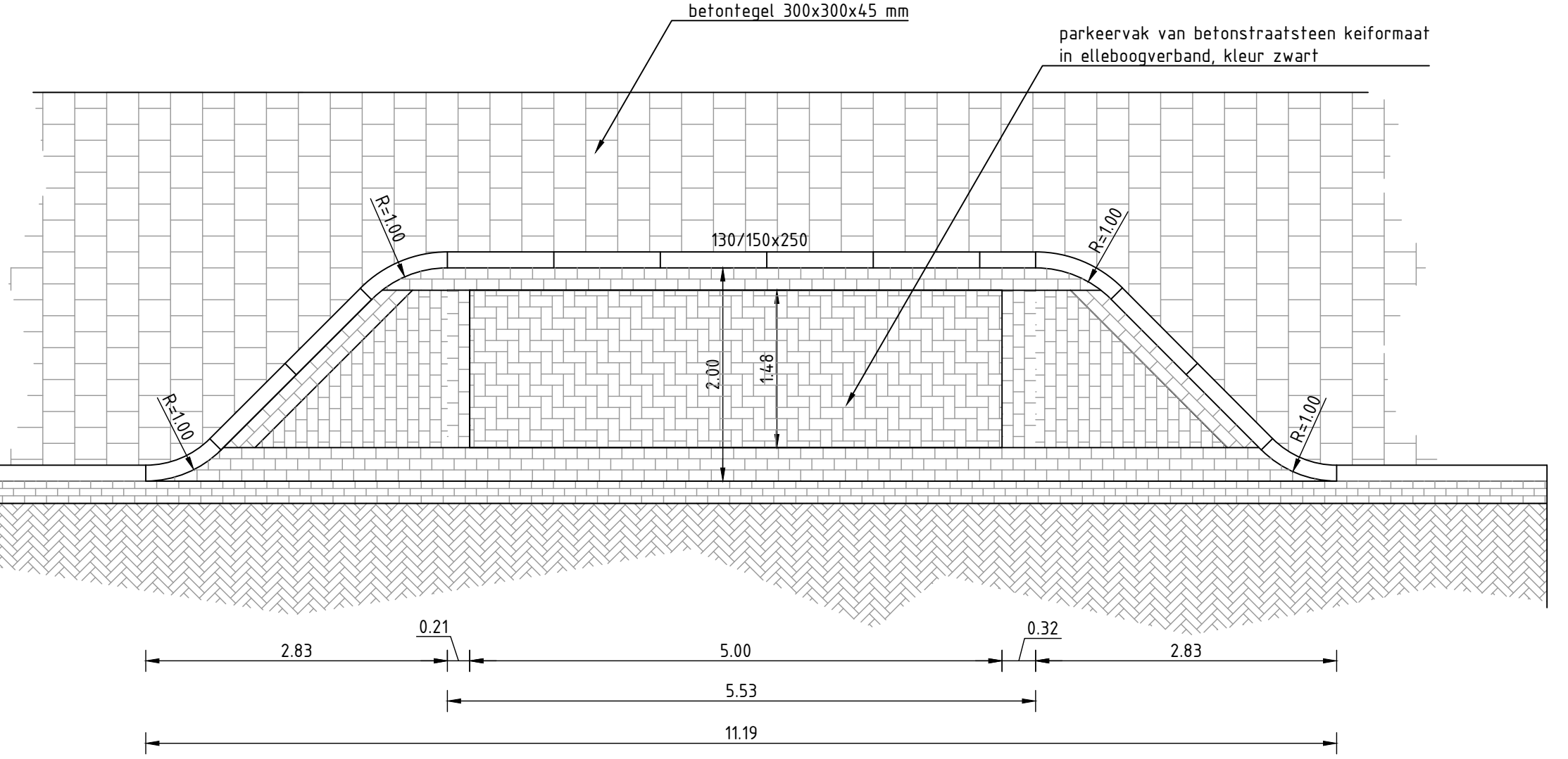
Principe langsparkeren Schaal 1:50
